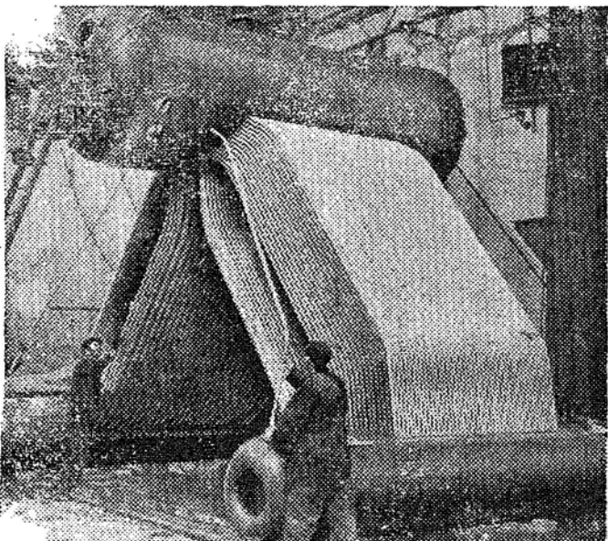
Na fotografia vemos a montagem da máquina Yarrow, nos estaleiros da Vickers-Armstrong em Barrow-in-Furness. - (B. N. S.)
