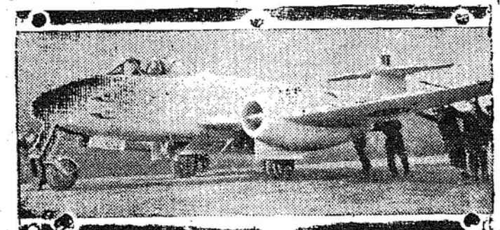
Esta é uma das primeiras fotografias do aparelho de propulsão a jato da RAF — o "Meteor". É um caça de um só lugar, acionado por dois motores Welland ou Derwent. Sua velocidade de aterrissagem não é muito grande e é altamente manobrável. O "Meteor" está armado com 4 canhões de 20mm. (Foto do BNS)
