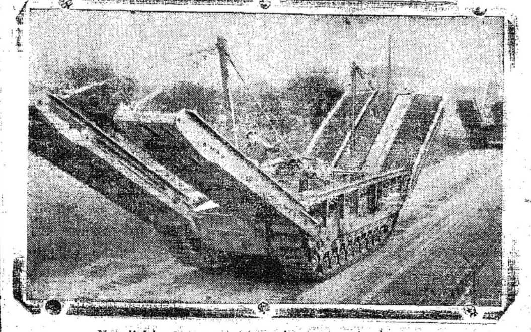
No clichê vê-se a estrutura de uma ponte de emergência. Acervo: Biblioteca Pública SC - Universidade Federal de Santa Catarina. (Foto do B.N.S.)
