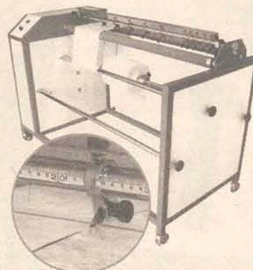
Máquina de refilar não tecidos para bordado
