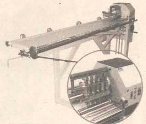
Máquina para cortar vize friso Semi-automática
