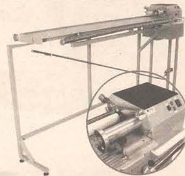
Máquina para cortar vize friso Semi-Automática
