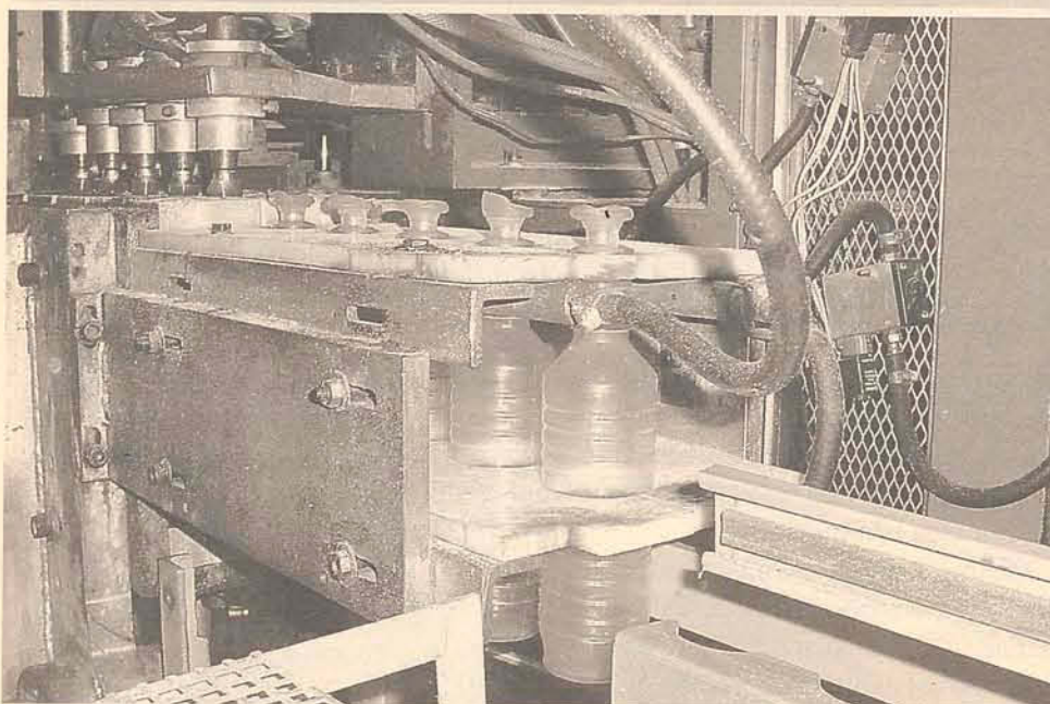
Garrafas são produzidas na máquina de sopro
