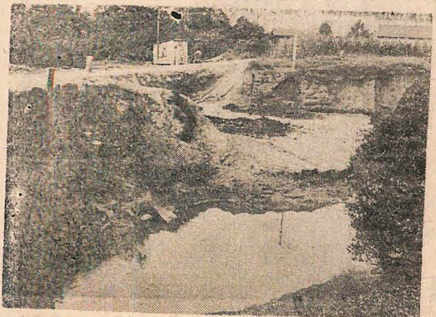
Ponte Gaspar Grande, em construção. Orçada em Cr$ 408 mil, Cr$ 208 mil de recursos próprios e Cr$ 200 mil da verba de auxílios para enchentes. Liga Gaspar a Gaspar Grande, Refúgio, Garuva e Gaspar Alto. Importante via de acesso e transporte de produção.
