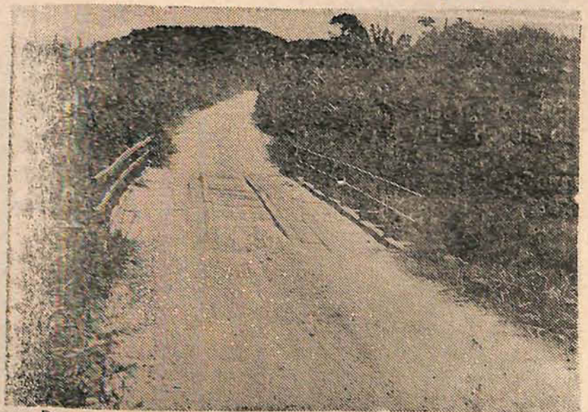
Ponte Belchior Baixo, mista, com fundamento de concreto. Liga Gaspar a Belchior Baixo, Central e Alto, Carolina, Alto Baú e Saltinho de Belchior. Escoação de produção abricular e industrial.
