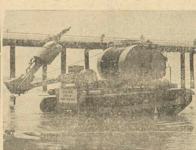
Na foto vê-se o aparelho chamado "Manipulador Subaquático de Controle Remoto", que é ligado por um cabo coaxial a um veículo em terra, sendo acionado por lagartas movidas eletricamente.
