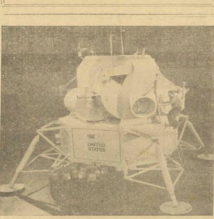
MÓDULO PARA EXCURSÃO LUNAR — Um técnico inspeciona um Módulo para Excursão Lunar destinado à nova expedição Apollo, na fábrica da Grumman Aircraft em Bethpage, Nova-Iorque. Os Estados Unidos designaram Apollo a seu programa de enviar três homens à Lua e traze-los de volta à Terra com o auxílio de um foguete Apollo. O dispositivo que se vê na foto possui 15 toneladas e se destina a transportar dois dos três astronautas do Programa Apollo da expedição Apollo à superfície da Lua para uma visita do 24 horas, levando-os de volta ao foguete espacial que os transportará de regresso à Terra. A Grumman construiu 20 módulos para provas em terra e em vôo a serem realizadas pela Administração Nacional de Aeronáutica e do Espaço (NASA).
