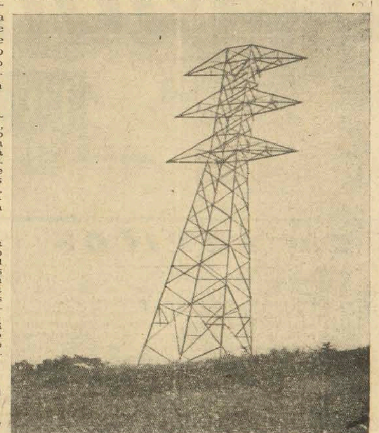
NA FOTO uma das 272 tórres de ferro perfildado que comporão o total de 104 km da "Linha Tronco Norte Joinville-Mafra", colocada nas proximidades do alto da Rua XV, em nossa cidade.
