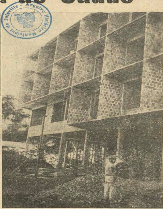
NO CLICHÊ um flagrante da nova edificação da Casa de Saúde "Dona Helena", notando-se alguns operários em pleno trabalho. A obra segue um ritmo normal de construção e deverá estar pronta dentro de um ano, aproximadamente.
