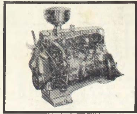
SUPER FORD F-600 — O mais moderno caminhão brasileiro. Construído para dar mais lucros em qualquer serviço... em qualquer estrada. Capacidade de carga: 6.500 kg. Motores: V-8, de 167 H.P. ou Diesel, de 128 H.P. Diferencial de 2 velocidades com reduzida elétrica, totalizando 10 marchas (8 à frente e 2 à ré). Distância entre eixos: 4,37 ou 3,76 m.
