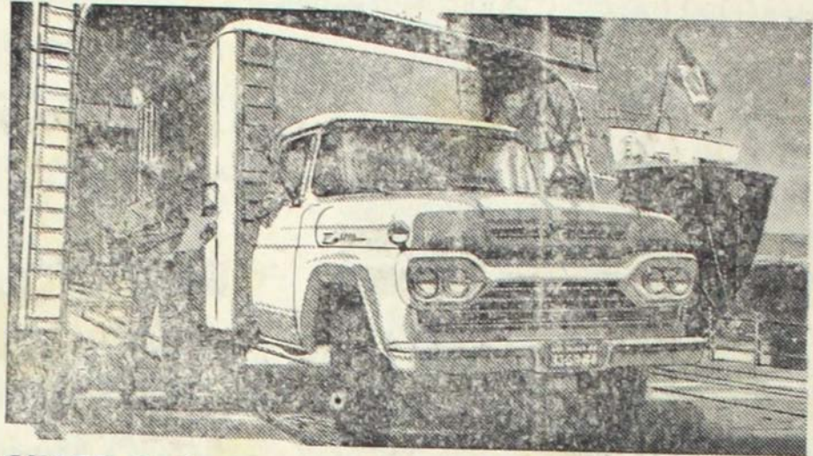
SUPER FORD F-350 — O único caminhão de tonelage média fabricado no Brasil, para o transporte de mercadorias relativamente leves, mas volumosas. Capacidade de carga: 2.670 kg. Motor V-8, de 167 H.P. Distância entre eixos: 3,30 m. Diferencial reforçado, tipo hipóide.
