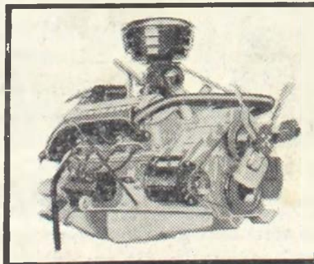
SUPER FORD F-600 — O mais moderno caminhão brasileiro. Construído para dar mais lucros em qualquer serviço... em qualquer estrada. Capacidade de carga: 6.500 kg. Motores: V-8, de 167 H.P. ou Diesel, de 128 H.P. Diferencial de 2 velocidades com reduzida elétrica, totalizando 10 marchas (8 à frente e 2 à ré). Distância entre eixos: 4,37 ou 3,76 m.
