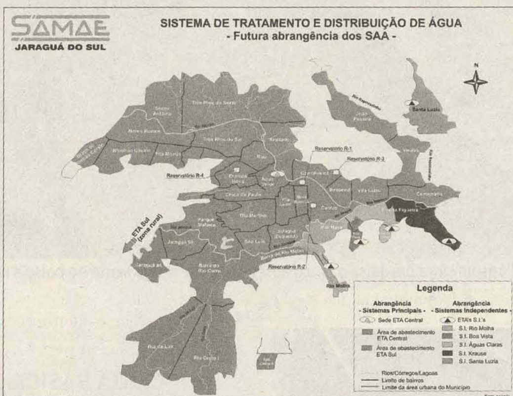
Mapas demonstram o abastecimento atual (acima), sem a ETA Sul, e a reconfiguração que acontece com a nova estação
