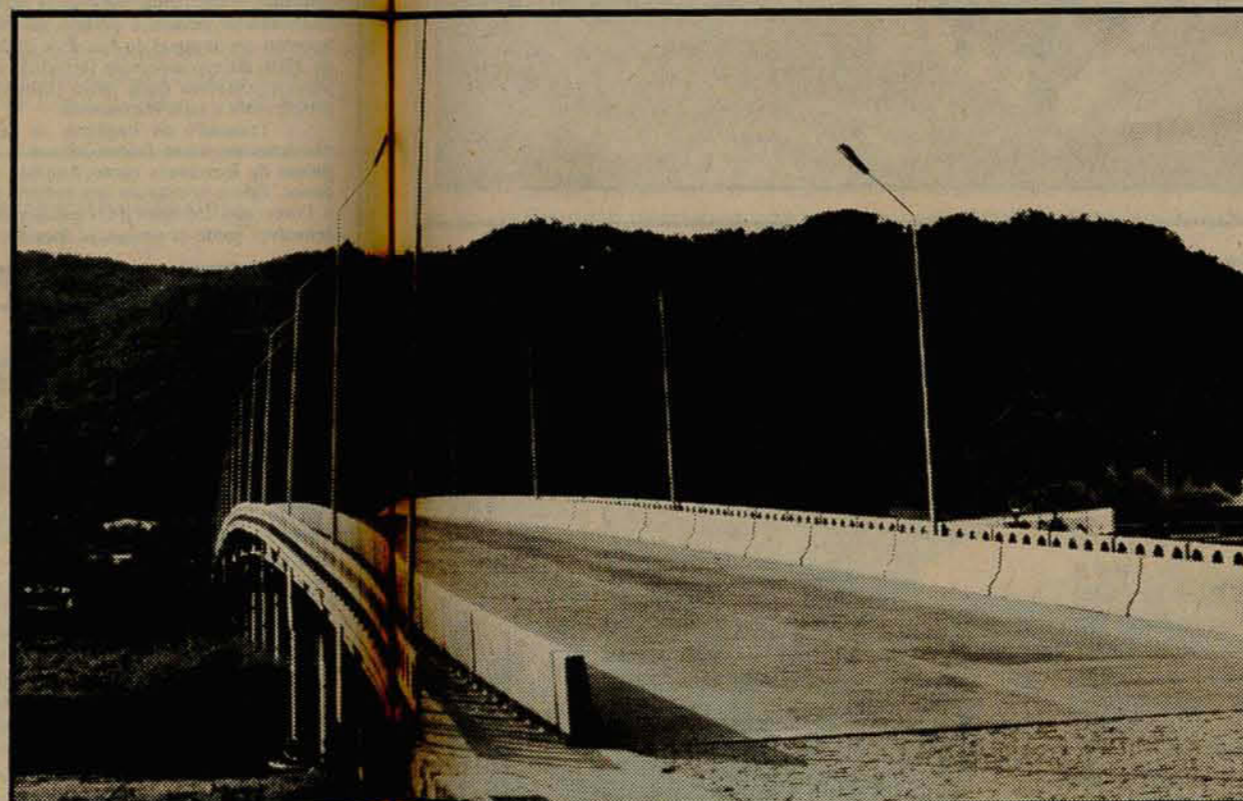
A maior ponte de Jaraguá do Sul, sobre o rio Itapocú, ligando os Bairros de Ilha da Figueira e Vila Lalau. Seu custo de construção alcançou 1,3 milhões de dólares, praticamente pagos com recursos próprios da municipalidade. A obra tem 223 metros de comprimento por 17 metros de largura.
