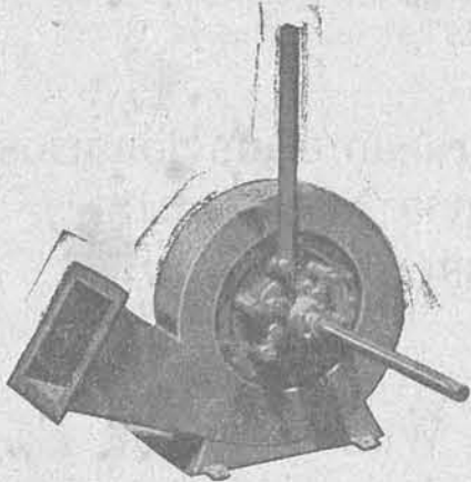
Turbina Hidráulica Tipo “Francis Espiral” marca MENEGOTTI
