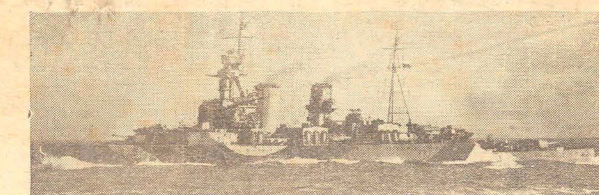
O "Frobisher" um cruzador do modelo do "Hawkins" possui armamento composto de sete canhões de 75 polegadas, quatro canhões anti-aéreos de 4 polegadas e 14 canhões menores, além de 21 tubos lança-torpedos. Deslocamento: 9,860 toneladas. Dimensões: 605 x 65 x 30.1j2. (BRITISH NEWS SERVICE)
